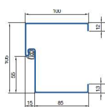
Ościeżnica blokowa 105/100
