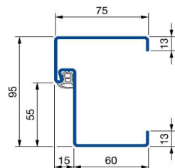
Ościeżnica blokowa 95/75
