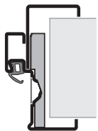
Ościeznica kątowa mocowanie diagonalne z zastosowaniem ościeznicy uzupełniającej Vario B53 C typ 1
