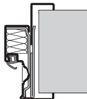
Ościeznica DryFix z ościeznicą uzupełniającą Vario B36 B-typ 2
