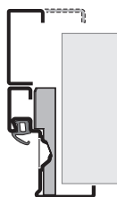
Ościeznica kątowa mocowanie diagonalne z zastosowaniem ościeznicy uzupełniającej C typ 2
