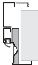
Eckzarge Diagonalbefestigung mit Ergänzungszarge C-Typ 2
