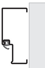
Ościeżnica blokowa typ 1 montaż w otworze E typ 1
