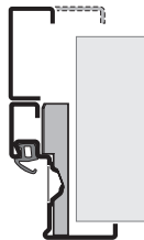
Ościeżnica kątowa mocowanie diagonalne z zastosowaniem ościeżnicy uzupełniającej C typ 2
