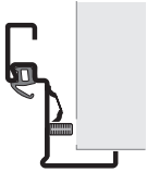
Ościeżnica kątowa mocowanie diagonalne (z zastosowaniem trzpieni gwintowanych) A typ 2
