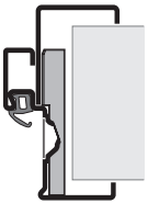
Ościeżnica kątowa mocowanie diagonalne z zastosowaniem ościeżnicy uzupełniającej Vario B53 C typ 1
