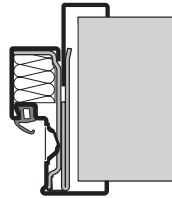
Ościeżnica DryFix z ościeżnicą uzupełniającą Vario B36 B-typ 2
