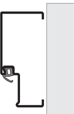
Ościeżnica blokowa typ 1 montaż w otworze E typ 1
