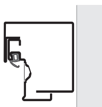
Ościeżnica blokowa 2-częściowa (z fabrycznie wykonaną okładziną) E typ 2
